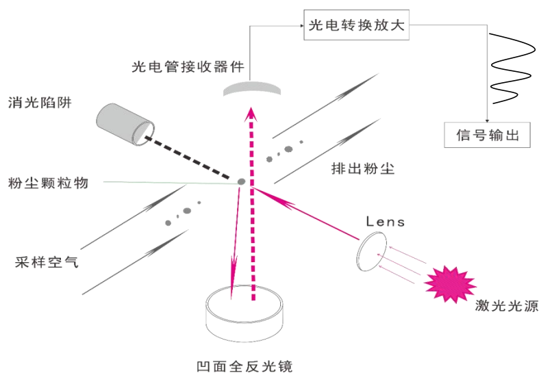
粉尘颗粒物激光传感器工作原理图
